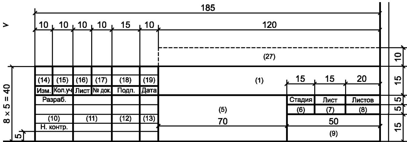
Рисунок И. 1– Форма и размеры основной надписи для пояснительной записки (первый лист ”Содержание”)
