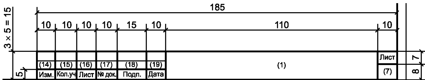
Рисунок И. 2– Форма и размеры основной надписи для последующих листов пояснительной записки и второго листа «Содержание»
